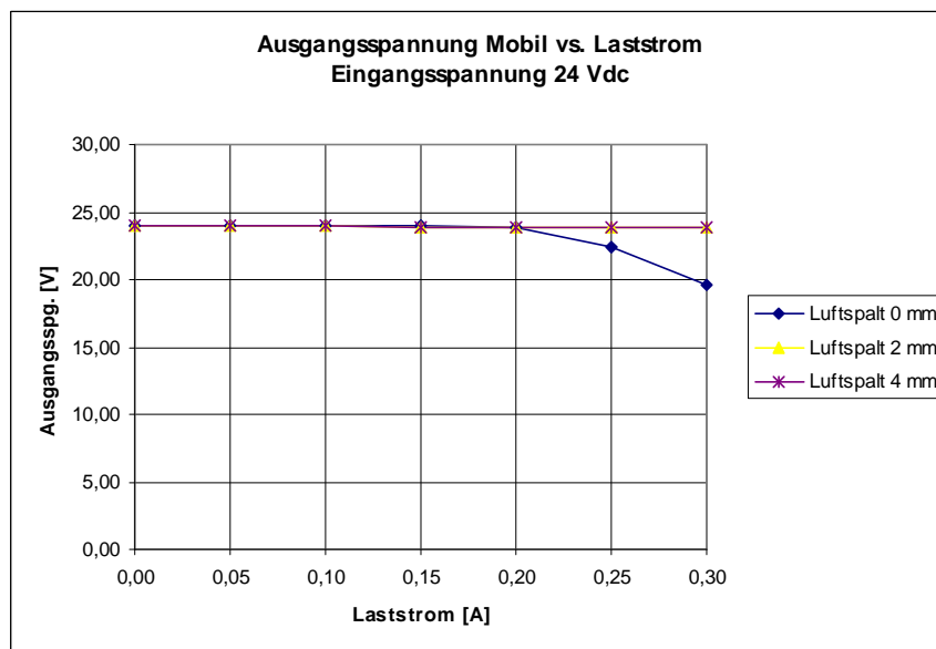
Bild 5 Lastcharakteristik Sensor Versorgung Mobil Einheit
