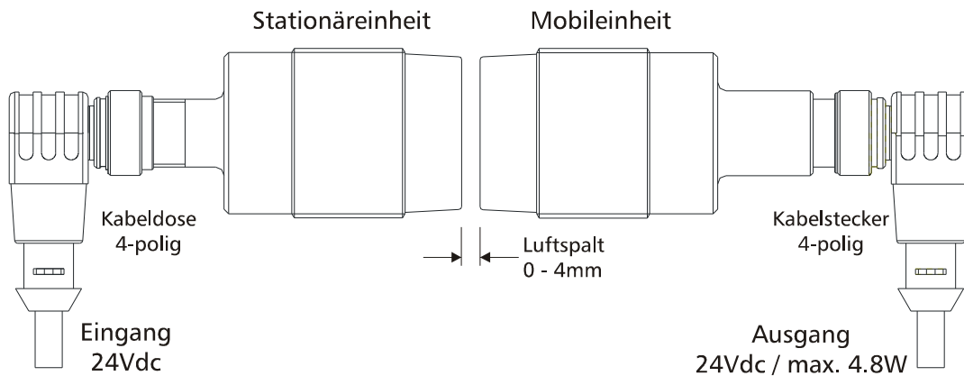
Bild 4 Module in Betriebsposition
